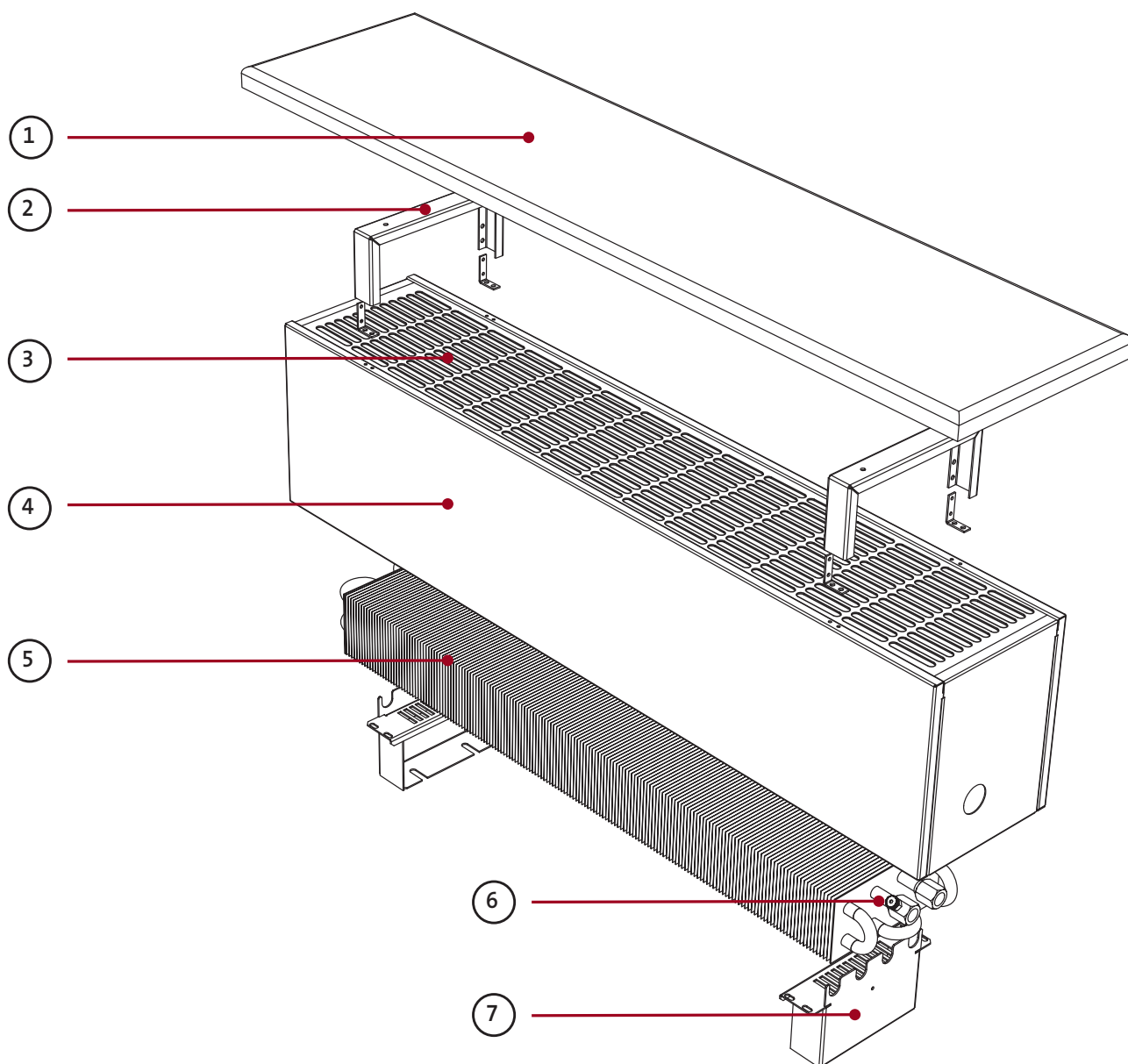
Устройство конвектора Aura Bench
